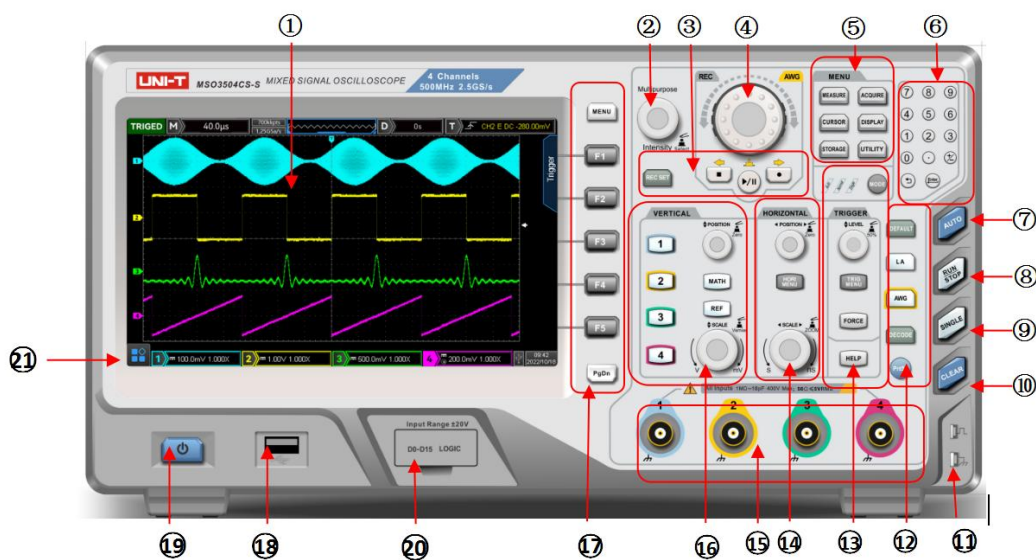
图 4-3 示波器前面板
